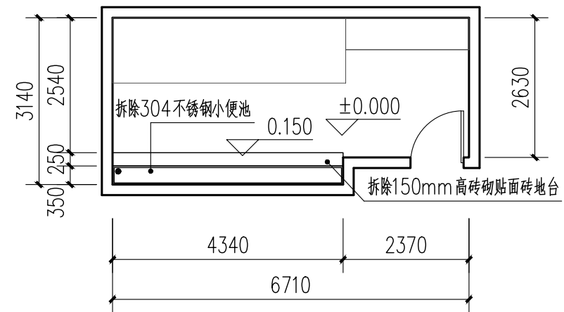
3号楼一至六层男卫平面图 1:100
