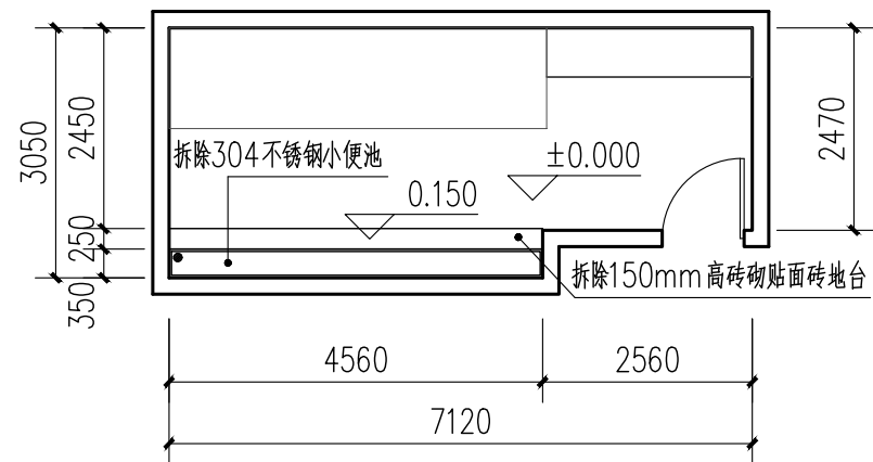
1号楼一至六层男卫平面图 1:100
