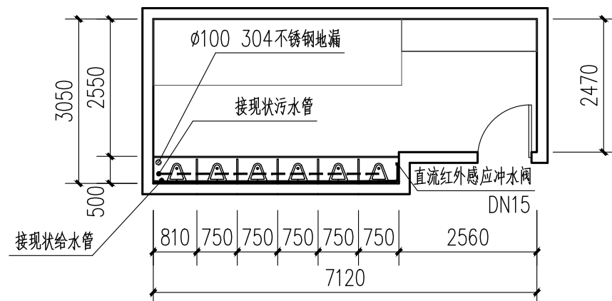
1号楼一至六层男卫给排水平面图 1:100
