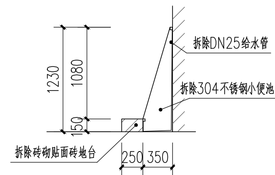
拆除小便池大样图
