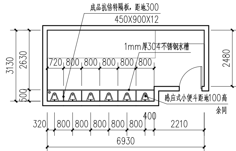
2号楼二至六层男卫改造后平面图 1:100
