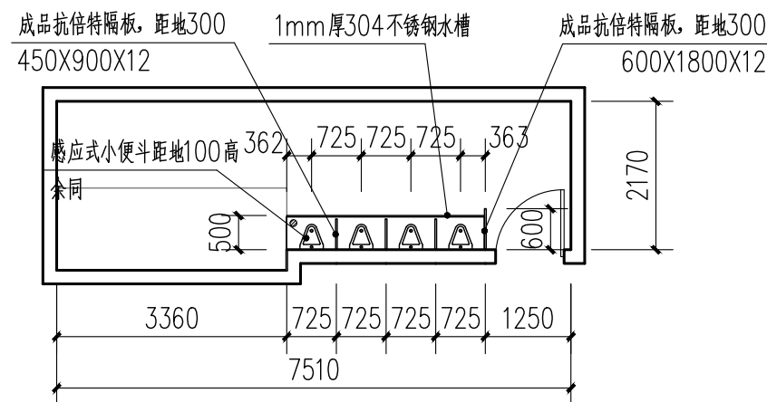
2号楼一层男卫改造后平面图 1:100
