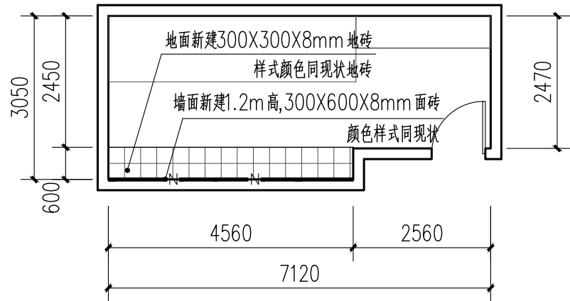
1号楼一至六层男卫改造后地面平面图 1:100
