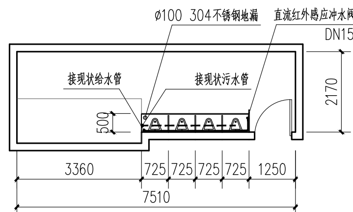
2号楼一层男卫给排水平面图 1:100
