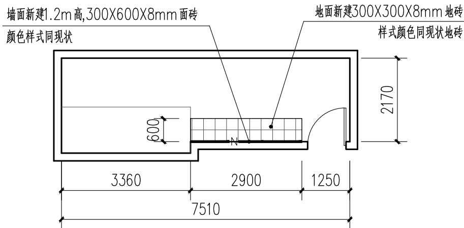
2号楼一层男卫改造后地面平面图 1:100
