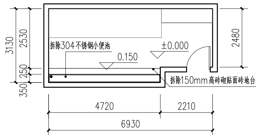
2号楼二至六层男卫平面图 1:100
