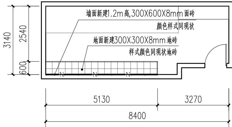
4号楼一层男卫改造后地面平面图 1:100
