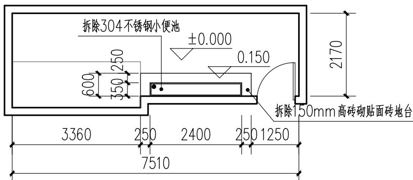
2号楼一层男卫平面图 1:100
