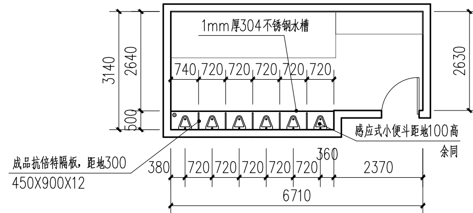
3号楼一至六层男卫改造后平面图 1:100
