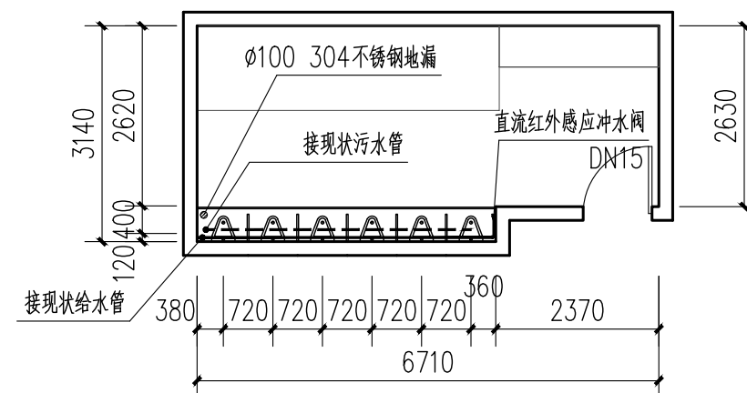
3号楼一至六层男卫给排水平面图 1:100
