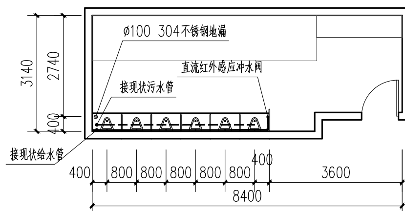
4号楼一层男卫给排水平面图 1:100
