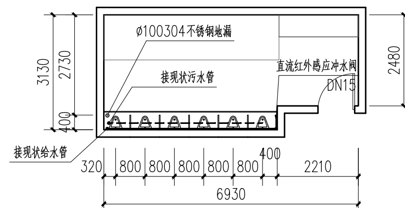
2号楼二至六层男卫给排水平面图 1:100
