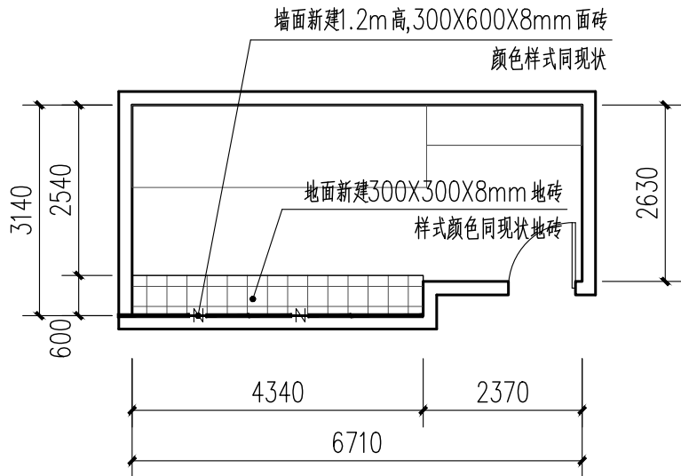
3号楼一至六层男卫改造后地面平面图 1:100
