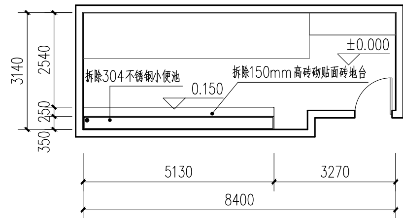
4号楼一层男卫平面图 1:100
