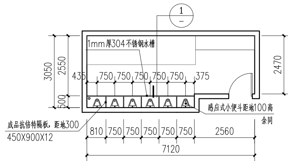
1号楼一至六层男卫改造后平面图 1:100
