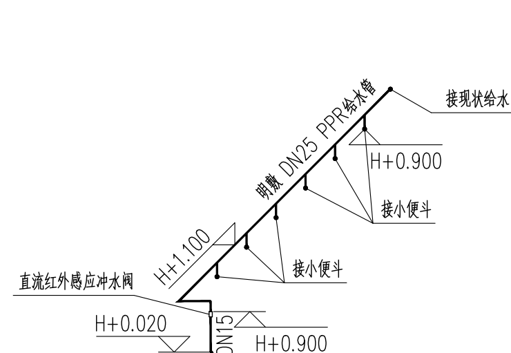
通用给水系统图 1:100
