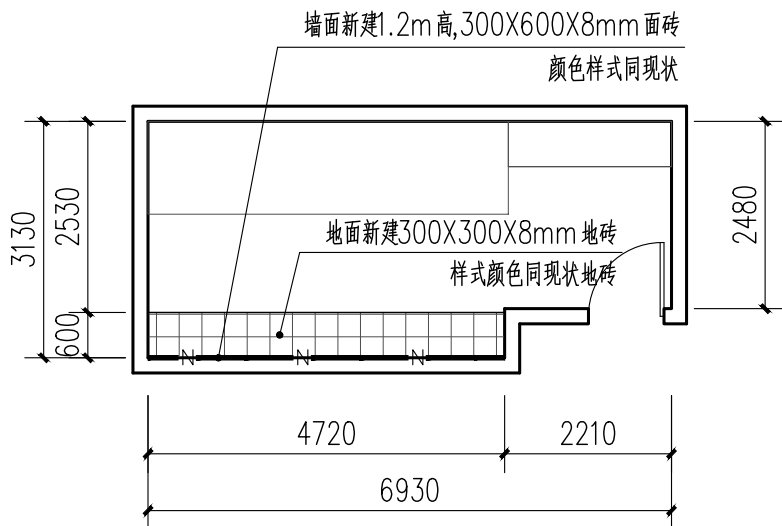
2号楼二至六层男卫改造后地面平面图 1:100
