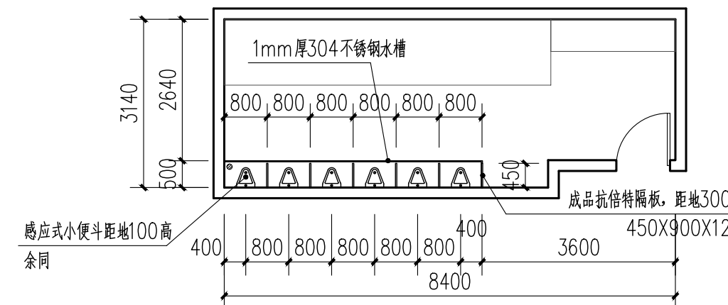
4号楼一层男卫改造后平面图 1:100
